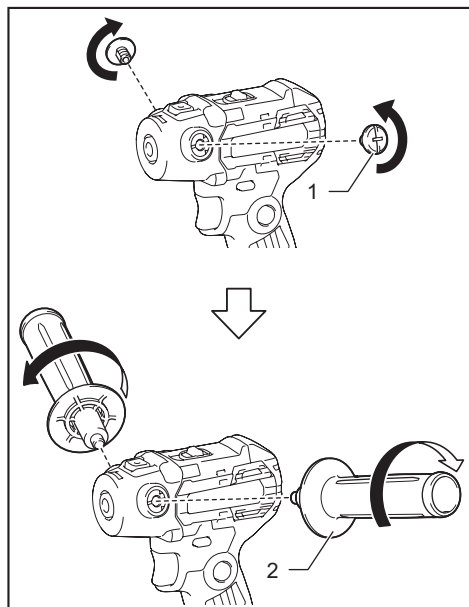
► 1. Bouchon 2. Poignée latérale
